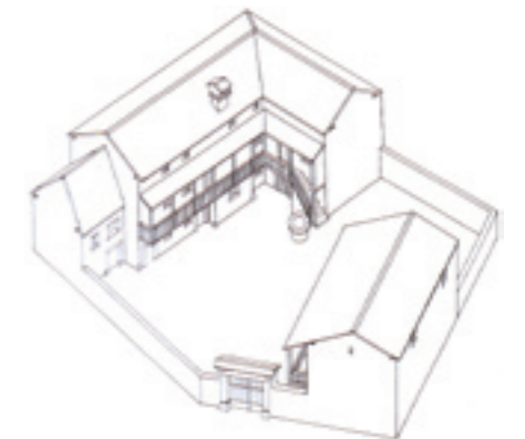
Shematicna rekonstrukcija razvoja značilnih prostorskih in oblikovalskih elementov kraške hiše. Vir: Ljubo Lah, Prenova stavbne dediščine na podeželju-KRAS, Tiskarna Novo Mesto 1994
